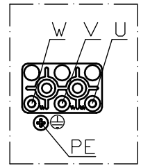
接线说明图
